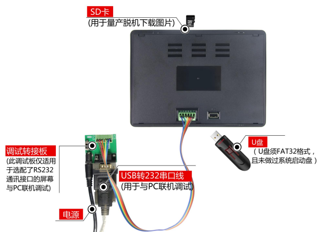
图 1-3 RS232 调试工具图
