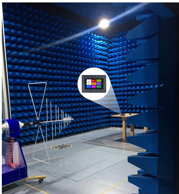
图 6-5 辐射测试图
