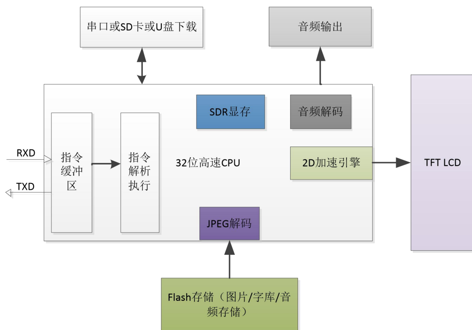
图 3-1 HMI 系列串口屏内部结构图
