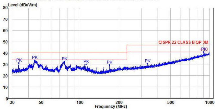
图 6-7 辐射测试垂直方向
