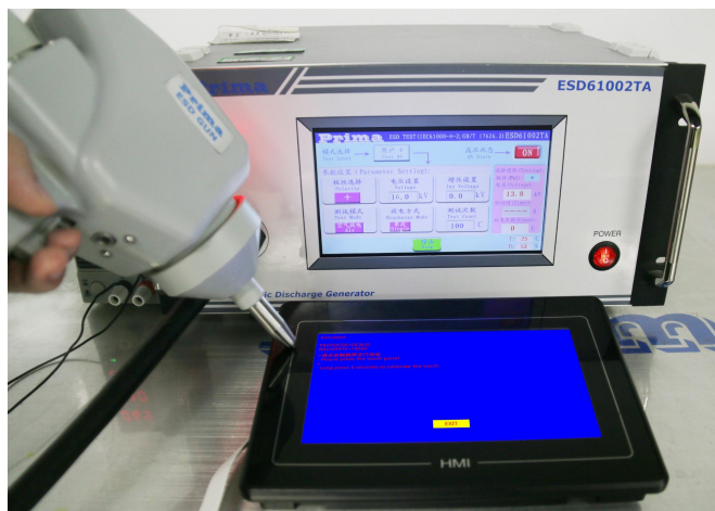
图 6-2 ESD 测试图
