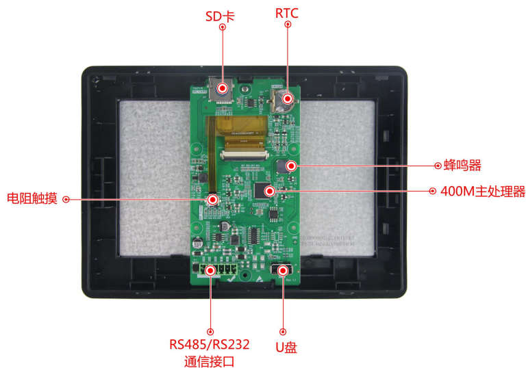
图 1-2 硬件配置图
